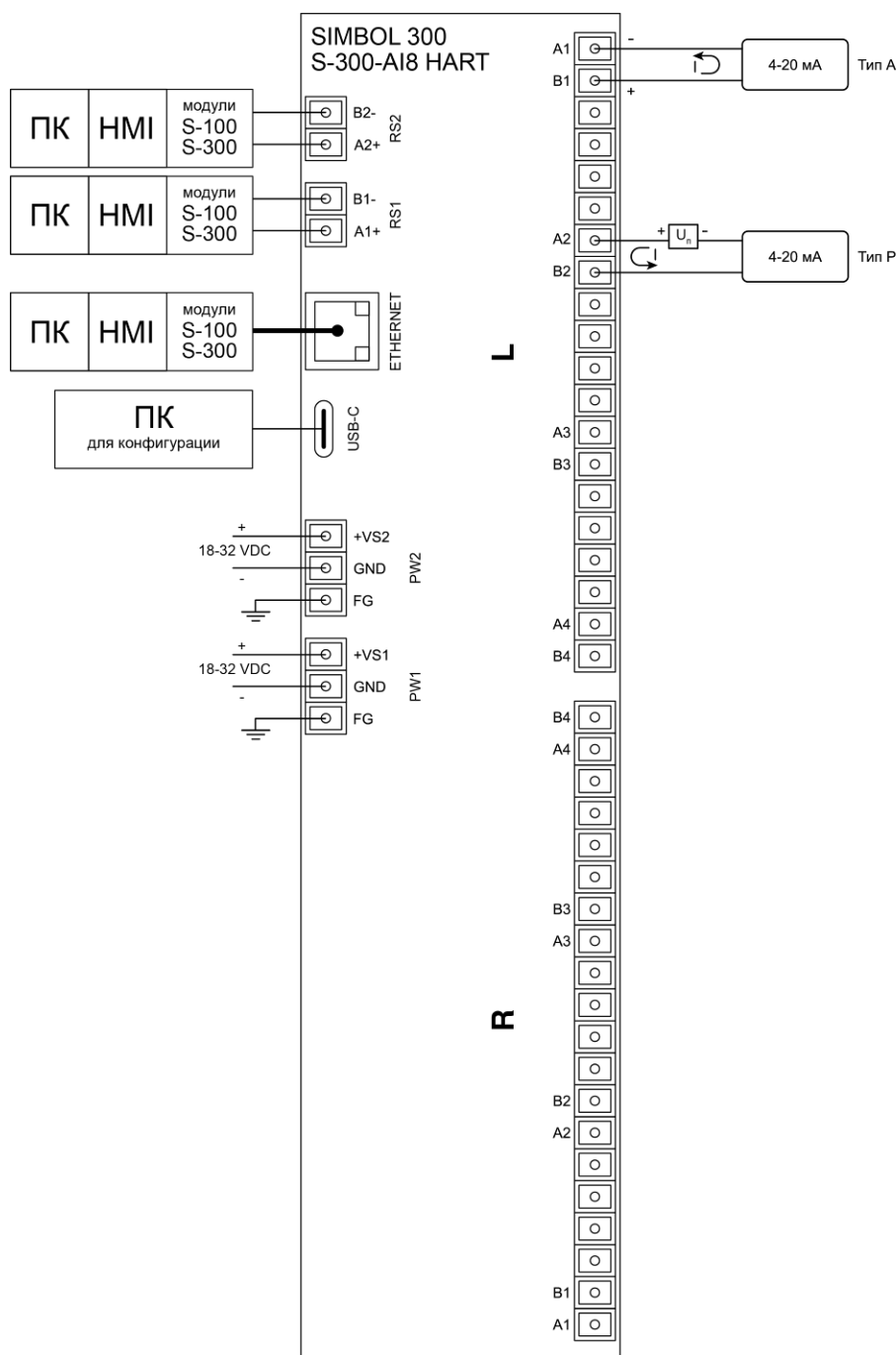
Рисунок 1.5 – Схема подключения модуля S-300- AI8 HART (S-300-AI4 HART)
